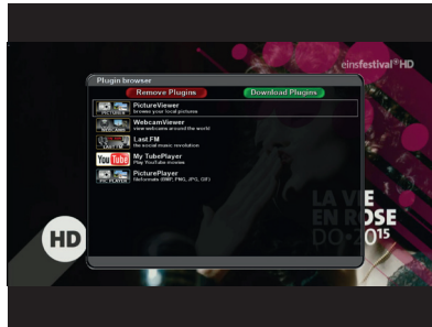
Plugin browser
